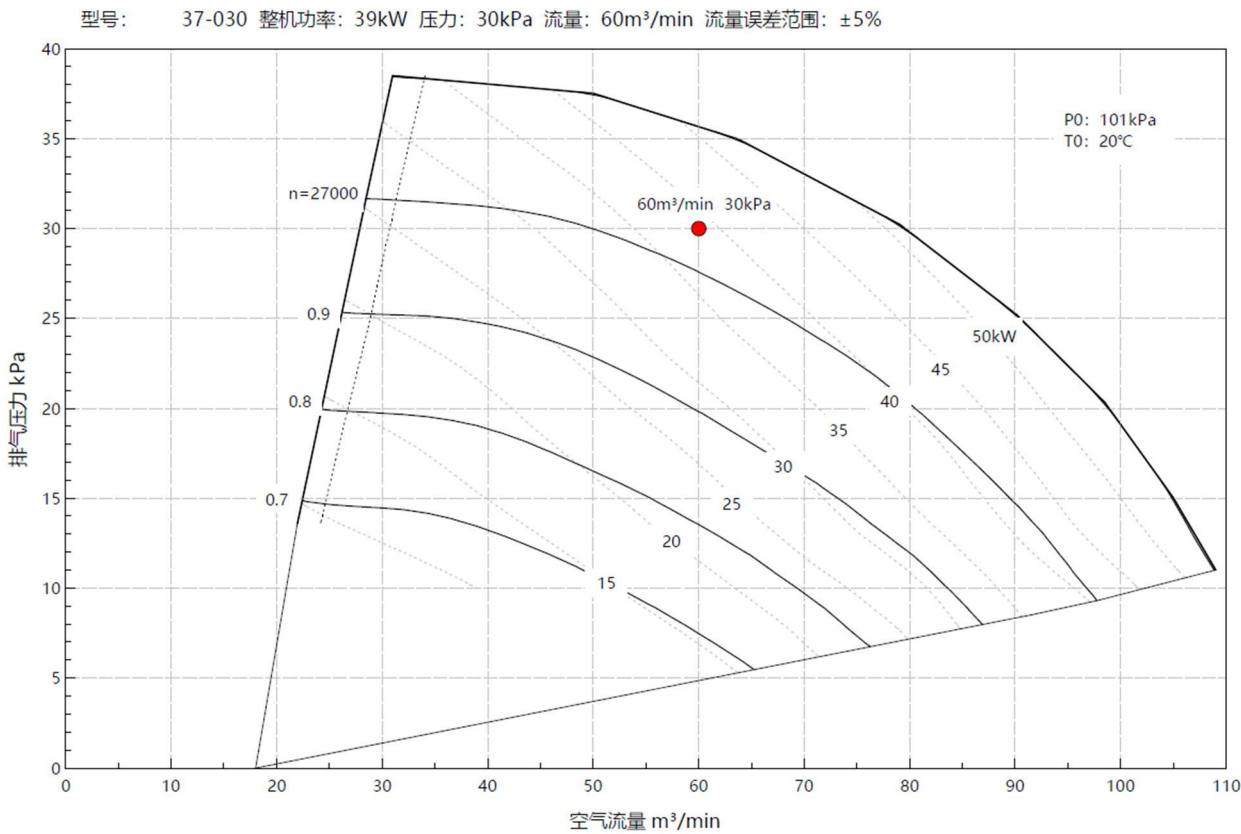
鼓风机性能曲线图
