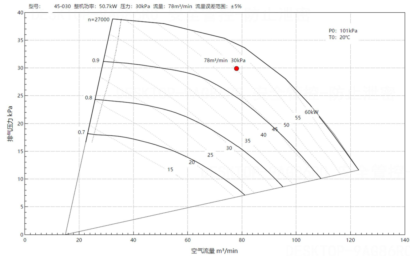
鼓风机性能曲线图
