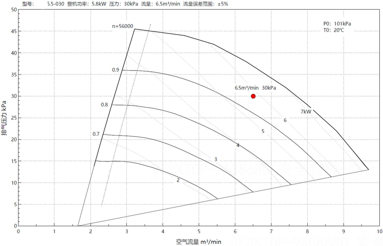
鼓风机性能曲线图
