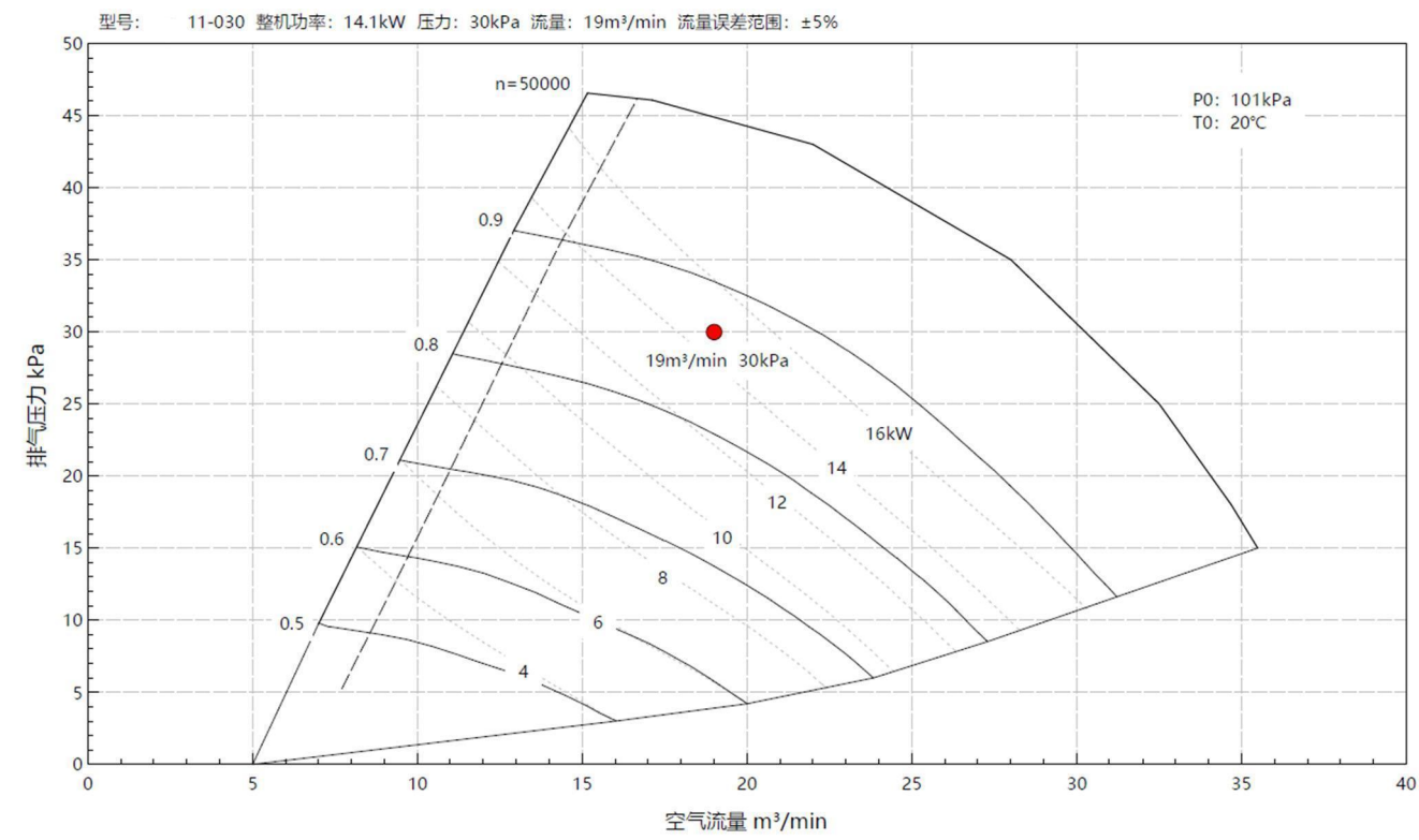
鼓风机性能曲线图
